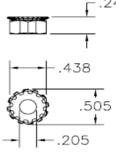
P/N 1000768 1/4 Kep Nut
