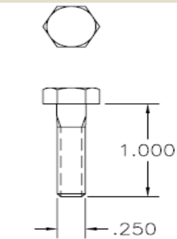
P/N 1000655 MS 1/4 x 1
